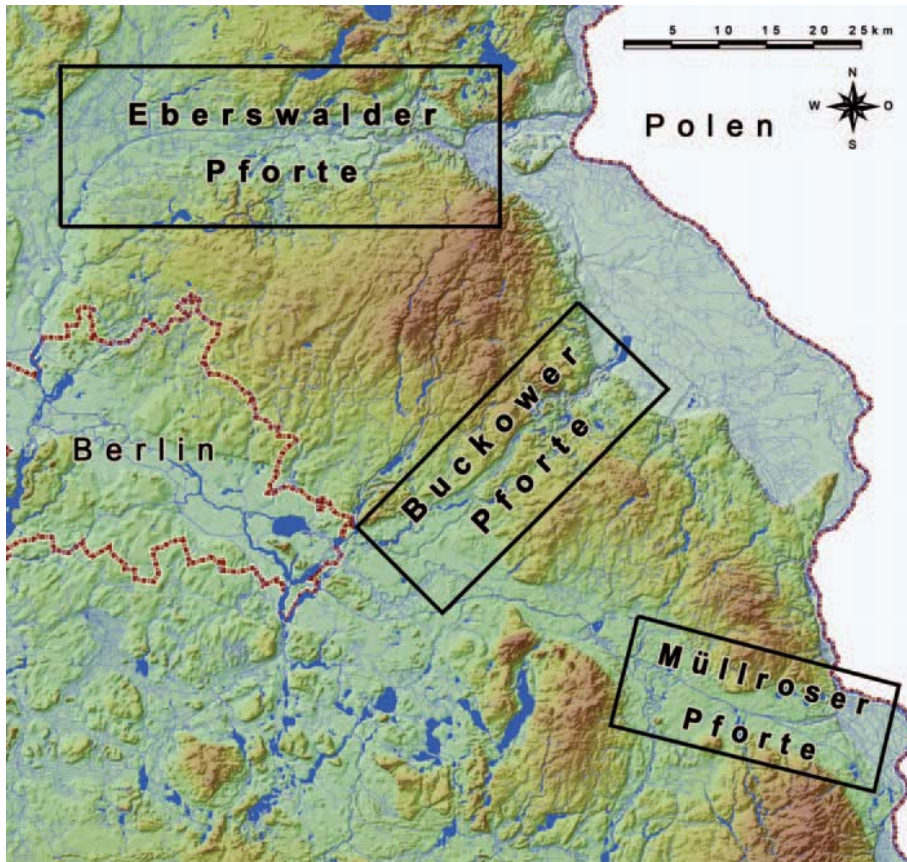
Abb. 11 Lage der Pforten potenzieller Flussanzapfungen von Elbzufüssen durch Nebenflüsse der Oder im Relieftext; basierend auf Daten des DGM 25, freigegeben durch die Landesvermessung und Geobasisinformation Brandenburg (LGB)
