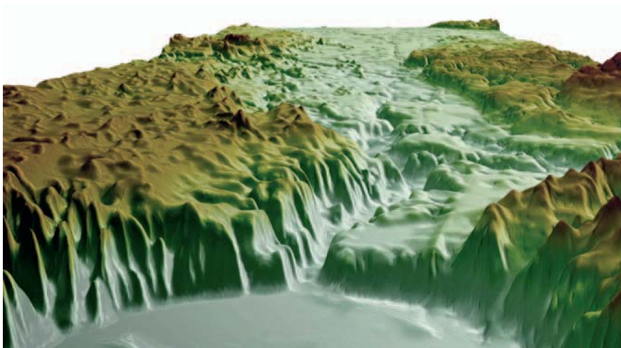
Abb. 6 Die Eberswalder Pforte; 3d-Darstellung mit Kerbtal des potenziellen Anzapfers Finow; Blick vom nördlichen Oderbruch nach Westen zum Haveltal (im Bildhintergrund von rechts nach links verlaufend); Darstellung 25fach überhöht, basierend auf Daten des DGM 25, freigegeben durch die LGB Brandenburg Fig. 6 The Eberswalde gate; 3d-display with gully of the potential piracy river Finow; View from northern Oderbruch to the west towards Havel valley (in the background from right to left); display exaggerated 25fold, based on data of DGM 25; courtesy of LGB Brandenburg
