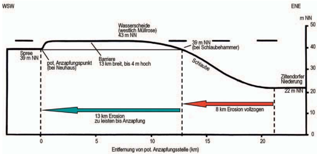
Abb. 7 Die Müllroser Pforte im Berliner Urstromtal; generalisiertes Querprofil
